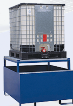
Typ: 6079/6079-Z Záchytná vaňa pre 1 IBC s roštom a možnosťou stáčania
