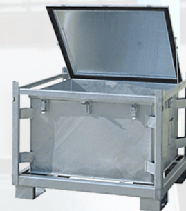
Typ 1255 Žiarovo-zinkovaný kontajner na tuhé nebezpečné odpady - 500 l - bez pogumovania
