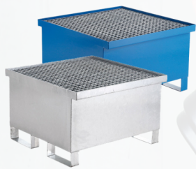
Typ: 7558/7558-Z Záchytná vaňa pre 1 sud s roštom
