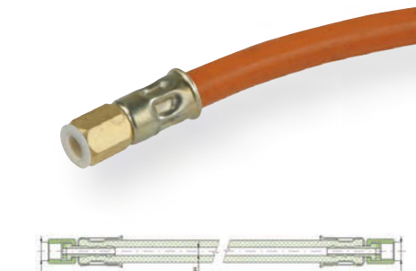
Hadica s koncovkami M9 x 0,75
