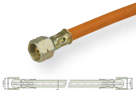
Hadica s koncovkami G 3/8 LH
