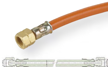
Hadica s koncovkami G 1/4 LH
