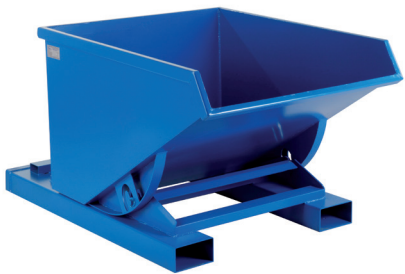
• 6502 Výklopný kontajner Profi Objem: 600 l Rozmery: 1650 x 1060 x 815 mm Materiál: oceľ Povrchová úprava: lak syntetika
