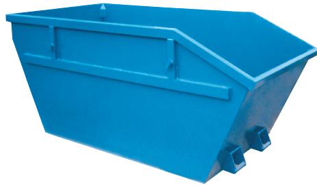
• 5602-1 Vaňový kontajner MULDA Objem: 5,5 m 3 do 10 m 3 Materiál: oceľ Povrchová úprava: lak syntetika
