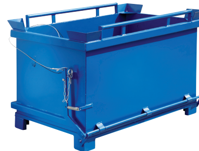
• 4727 Kontajner s výklopným dnom Objem: 1000 l Rozmery: 1500 x 1080 x 970 mm Materiál: oceľ Povrchová úprava: prášková farba
